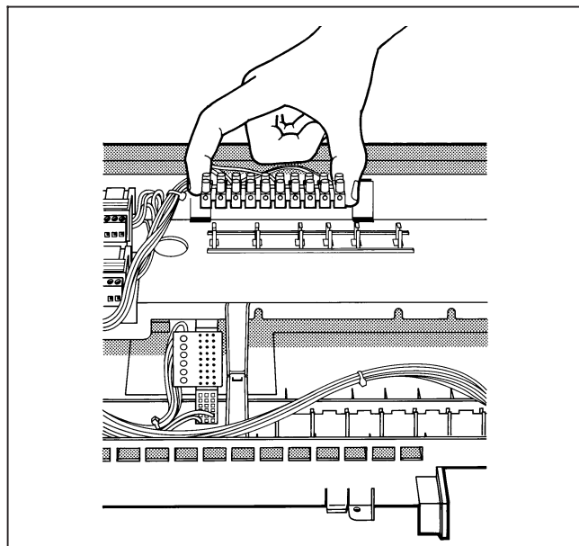
Рис. 4: насадить зажимы
