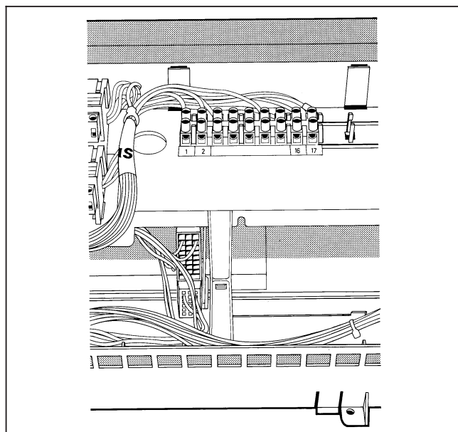
Рис. 5: наклеить наклейку
