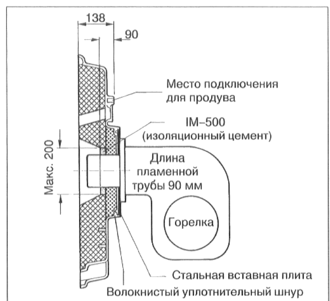
Рис. 25: Дверца горелки
