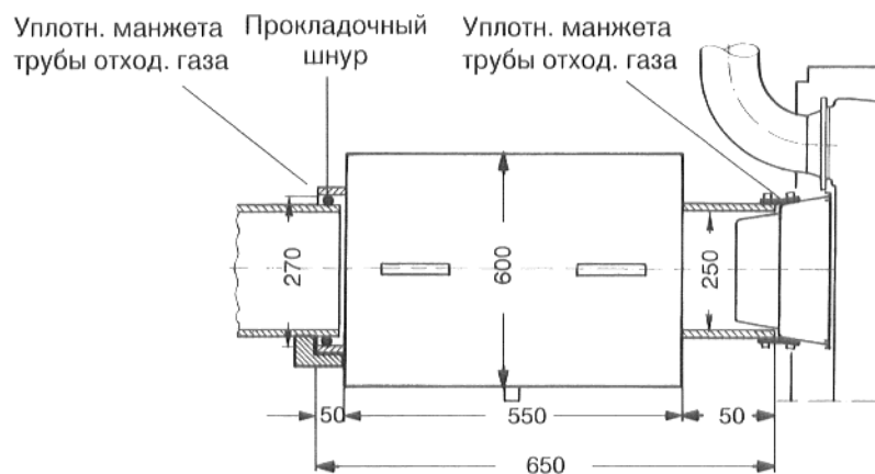
Рис. 61: звукопоглощающее устройство отходящего газа
