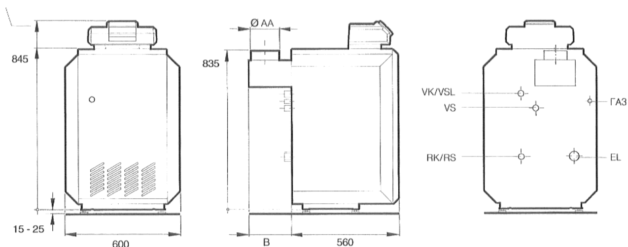
Рис 1: вид спереди, сбоку и сзади - G124 X
