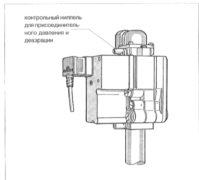
Рис. 30: арматура газовой горелки "BM" 762-012
