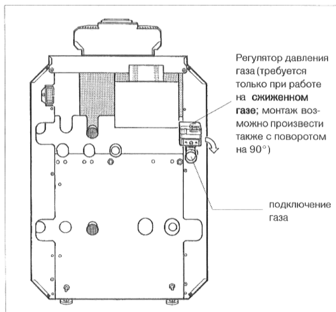
Рис. 23: подключение газа
