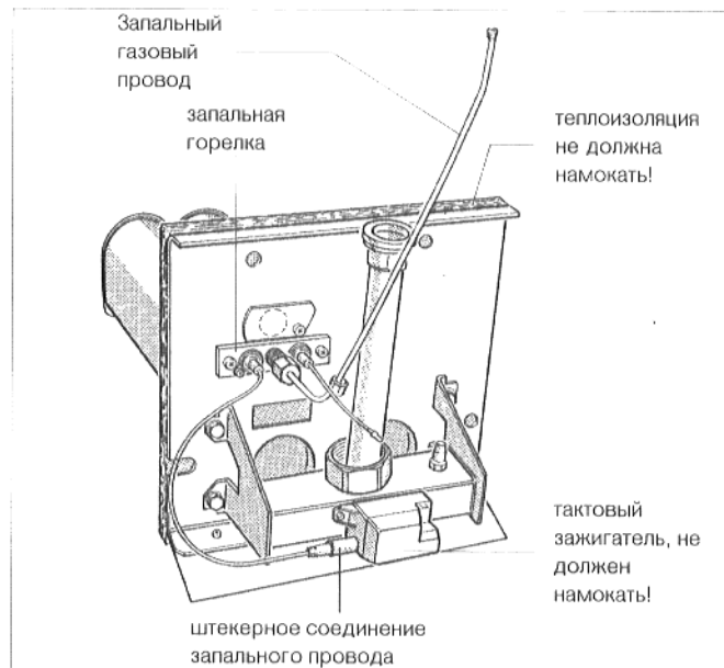
Рис. 46: газовая горелка
