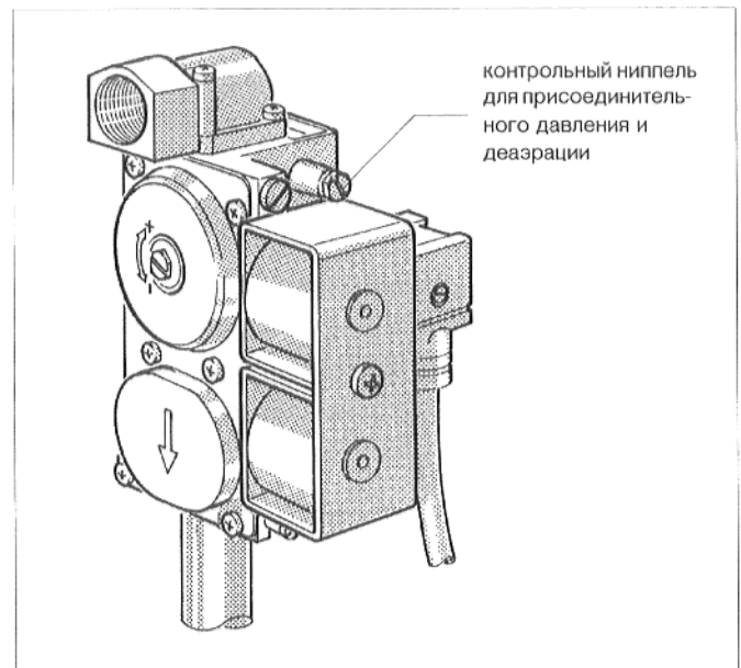
Рис. 29: арматура газовой горелки "SIT" 830 Tandem
