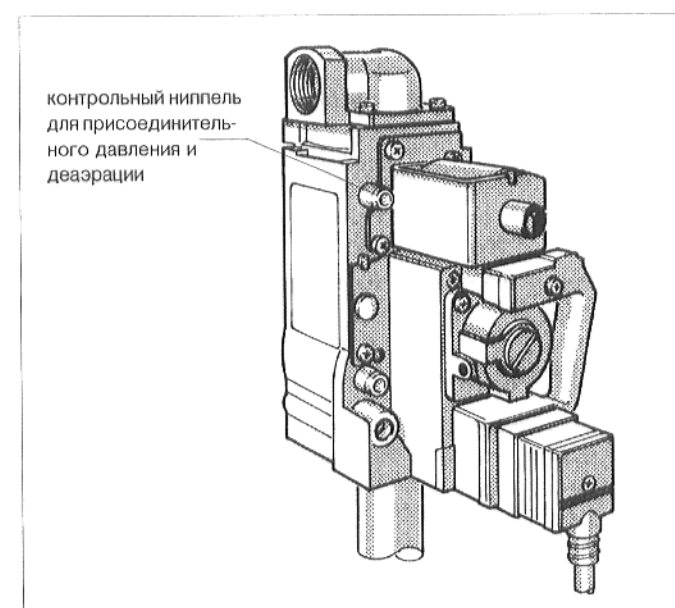
Рис. 31: арматура газовой горелки "Honeywell" VR 4601
