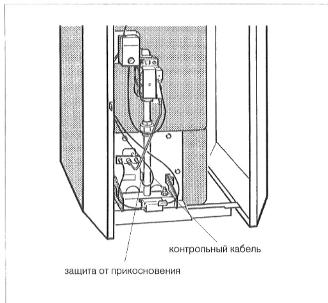
Рис. 34: контрольный кабель
