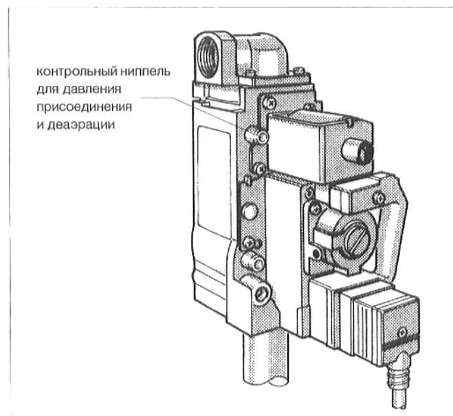
Рис. 25: арматура газовой горелки "Honeywell" VR 4601
