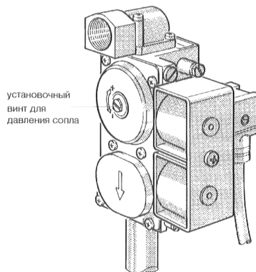
Рис. 53: газовая арматура "SIT" 830 Tandem
