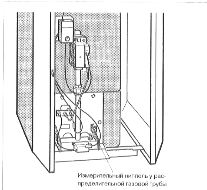
Рис. 32: газовая горелка
