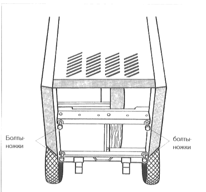
Рис. 5: котел снизу
