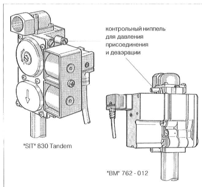
Рис. 24: "SIT" 830 Tandem и "BM" 762 - 012
