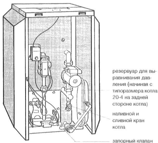
Рис. 9: G124 XV, передняя стенка открыта
