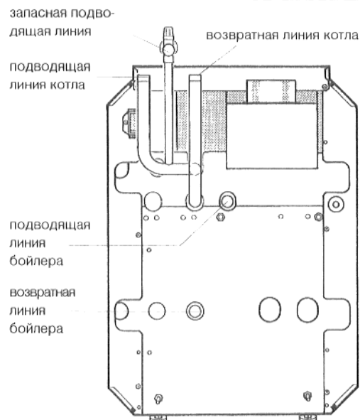
Рис. 8: подключение воды G124 XV
