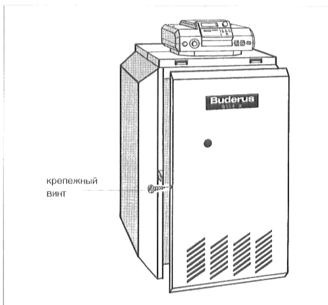
Рис. 37: монтаж передней стенки котла
