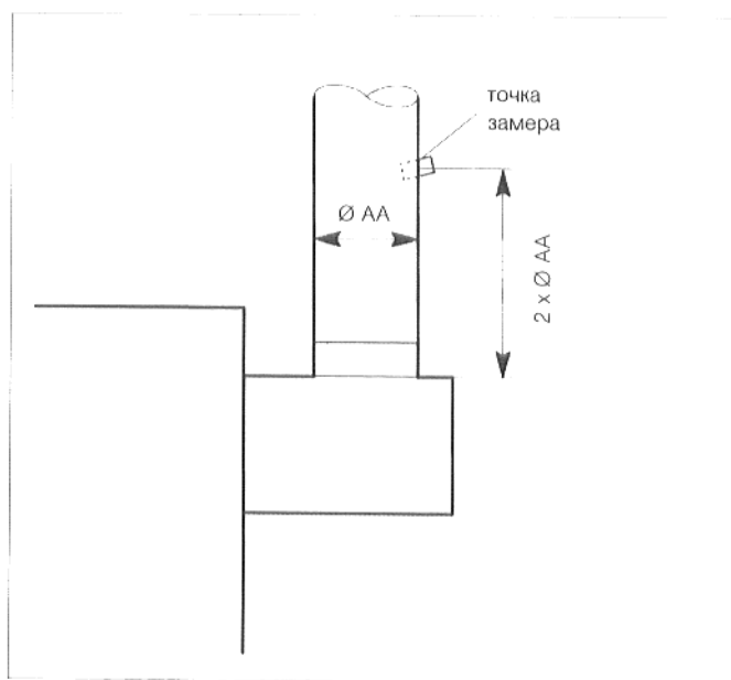
Рис. 33: точка замера в трубе отходящего газа
