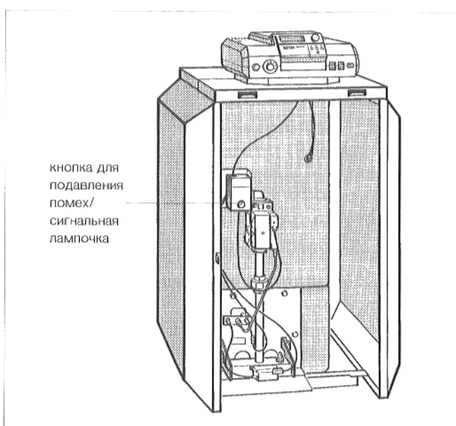
Рис. 28: кнопка для подавления помех
