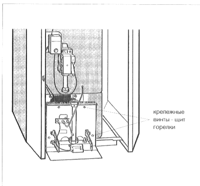
Рис. 43: демонтаж горелки
