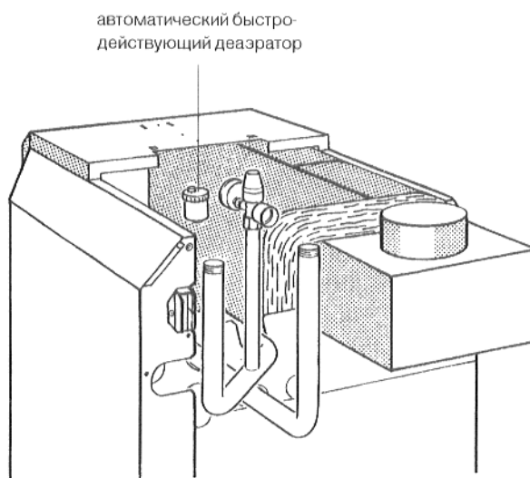
Рис. 10: автоматический быстродействующий деаэратор G124 XV
