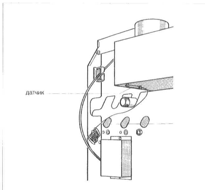
Рис. 36: датчик контроля отходящего газа
