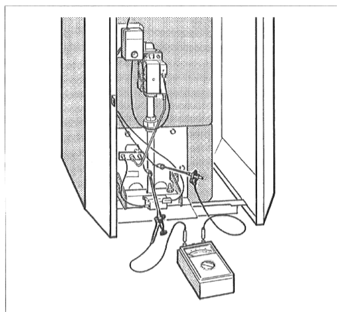
Рис. 35: замер ионизационного тока
