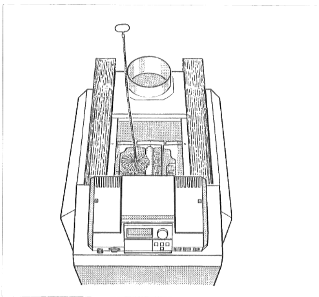
Рис. 44: очистка щетками
