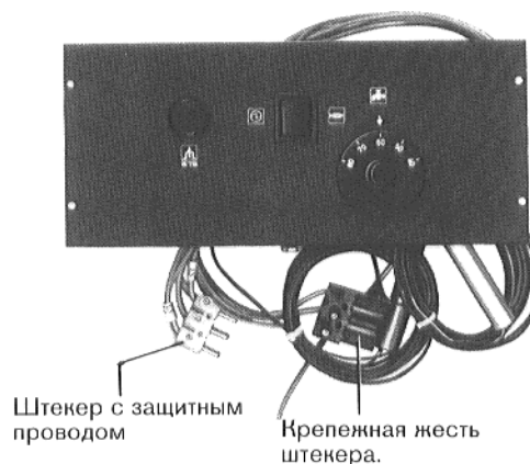
Рис. 8 – модуль S 102
