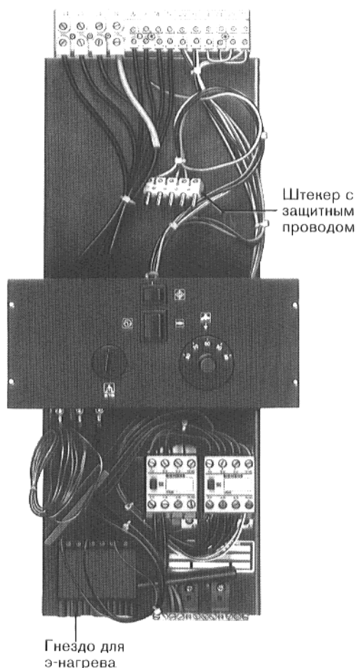
Рис. 10 – Модуль S 106/109
