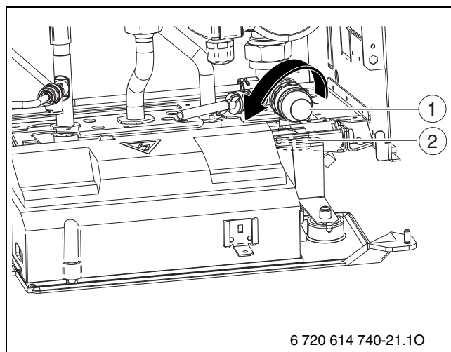
Рис. 37 Предохранительный клапан
