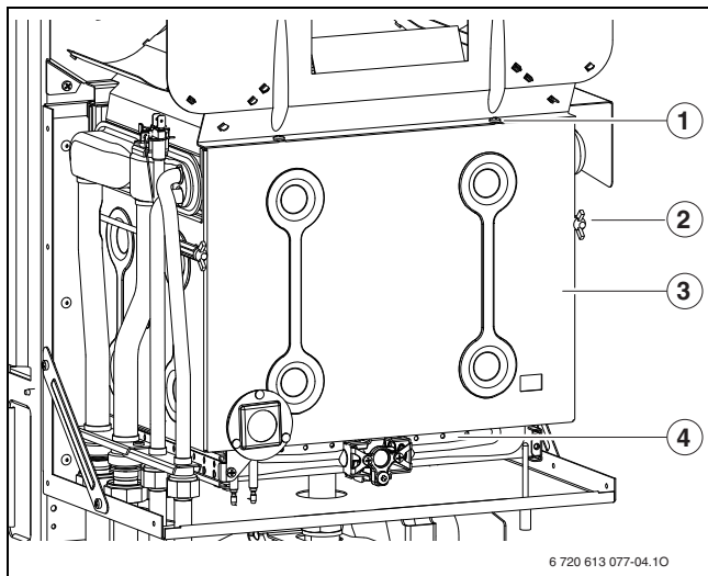
Рис. 30 Открывание горелки
