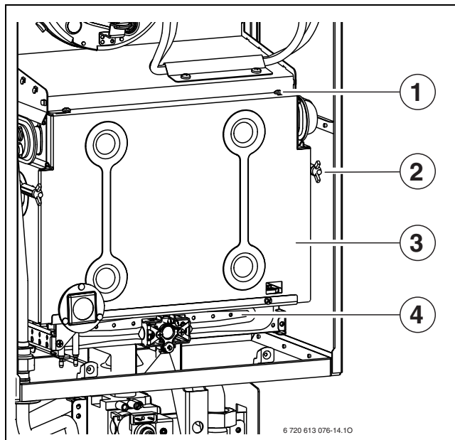
Рис 34 Открывание горелки
