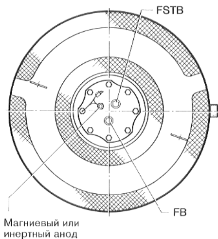
Рис. 3 Вид сверху ST 301 D/F – ST 951 D/F
