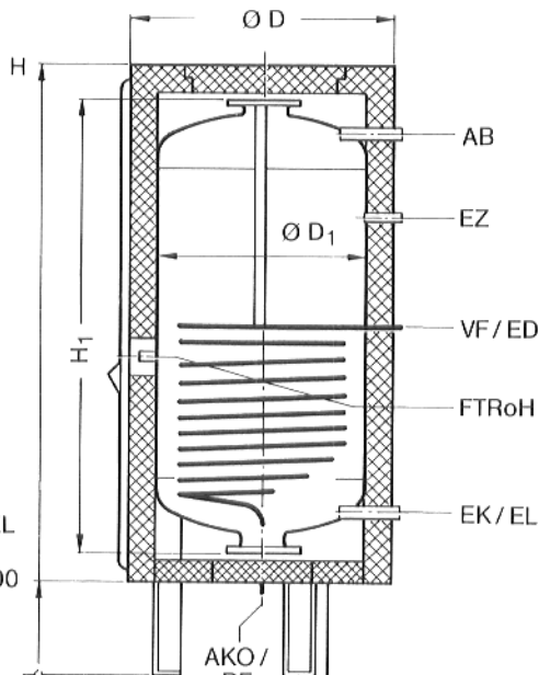
Рис. 2 ST 401 D/F – ST 951 D/F
