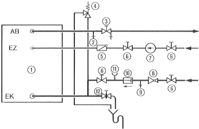
Рис. 10 Схема установки бойлер-нагреватель хозяйственной воды „TBS-Isosol„
